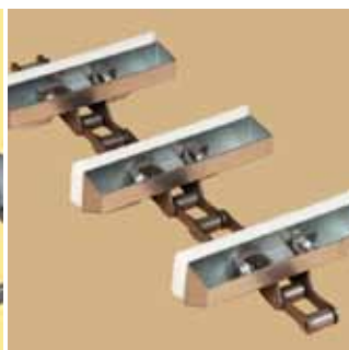
Chaîne avec godets de retour.
